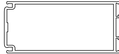
C057 Wide Pivot Stile
